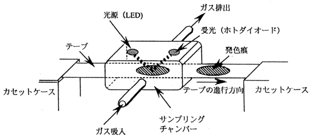
構造図
